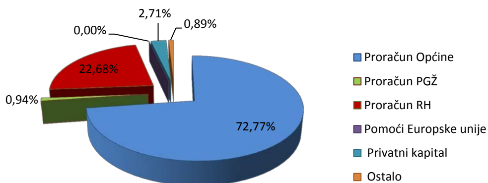
Grafikon 4: Ukupno ostvareni izvori sredstava za realizaciju mjera/projekata u 2015. godini
